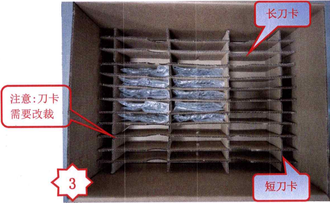
图三, 将 PA2629 按照每层 30PCS, 每箱 2 层的方式进行包装, 同时在底层和每层的顶部放一块隔板, 共 3 块隔板。
